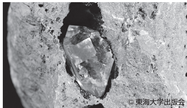
図5：石英（ハークマー水晶；アメリカ合衆国ニューヨーク州産）ニューヨーク州ハークマーで採れる石英。短柱状で両端の尖った形を示す。非常に透明度が高く、結晶面の光沢が強いので、ハークマーダイヤモンドとも呼ばれる。
