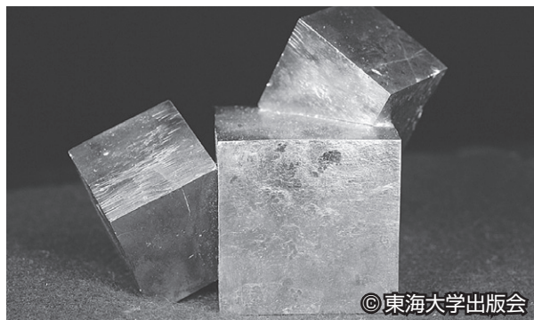
図3：黄鉄鉱（スペイン共和国・リオハ州産）
