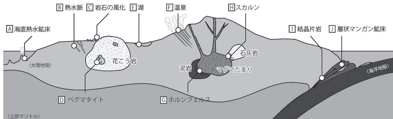
図1：鉱物が育つ場所（参考 株式会社小学館発行「小学館の図鑑NEO 10 岩石・鉱物・化石」）
