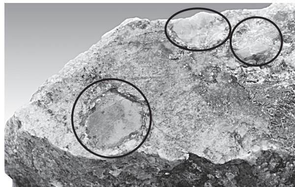
図14：コランダム（南砺市利賀村産）写真中の丸の部分
