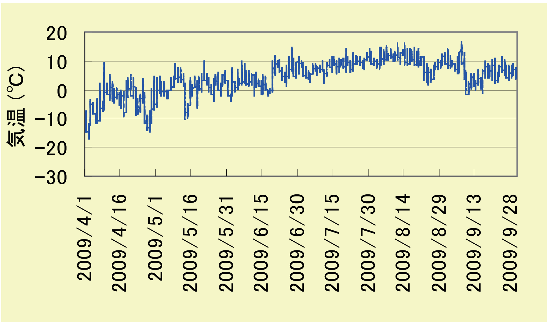
図1-15 浄土山山頂の春から夏の気温
