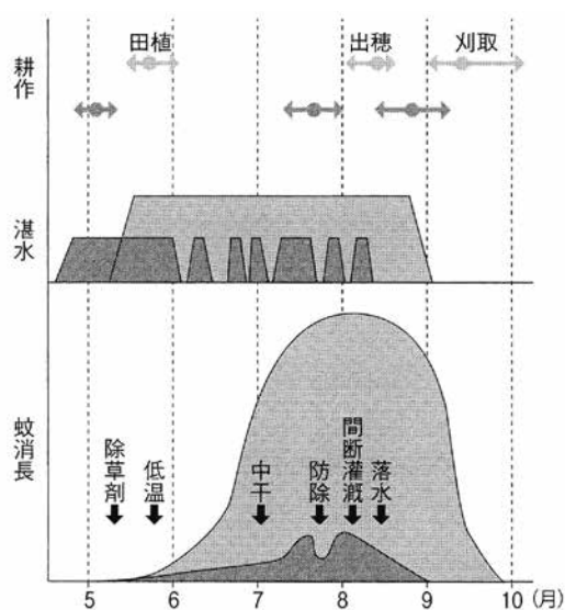
図6 稲作形態とコガタイエカ季節消長の変遷 (上薄い領域: 1950年、下濃い領域: 1975年)
