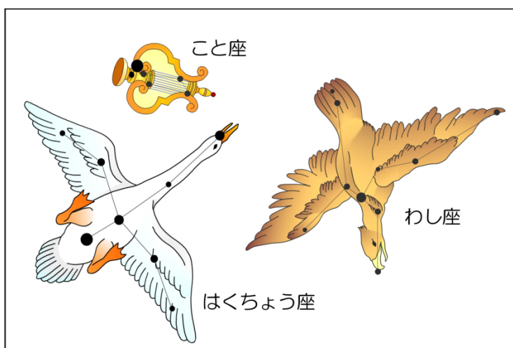
夏の大きな三角形の星座
