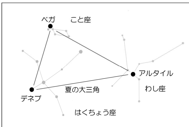
夏の大きな三角形の星々
